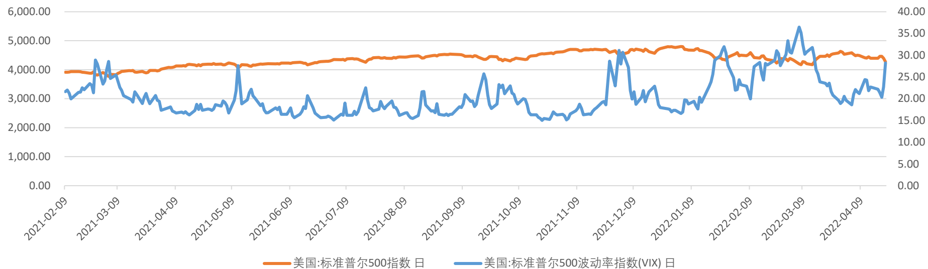
标普波指
