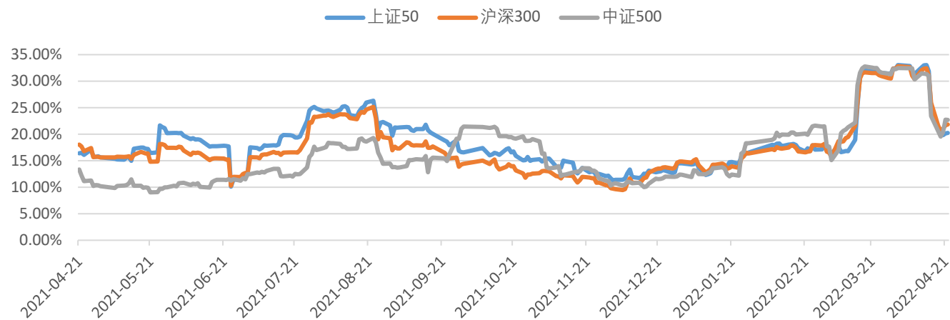
指数波动率
