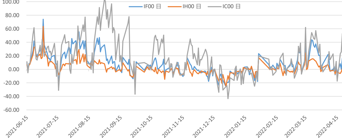
基差表现
